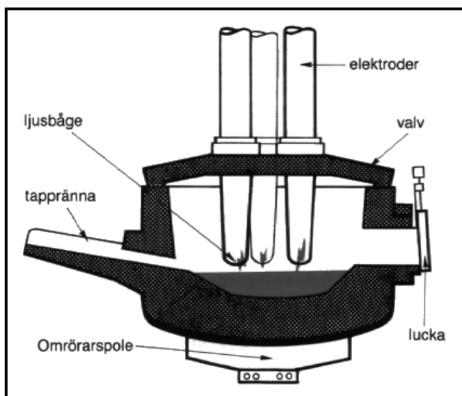
Figur 1 Ljusbågsugn
