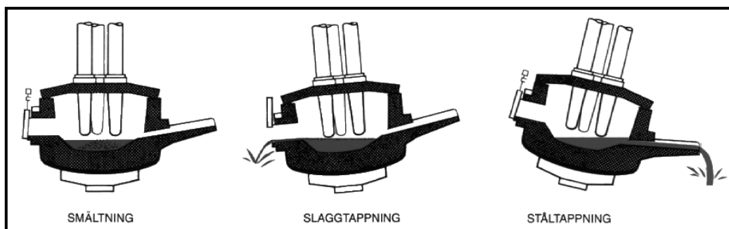
Figur 2 Tippbar ljusbågsugn
